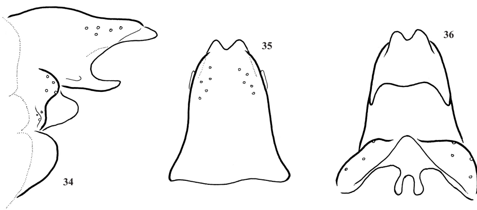
Figs 34–36. Chaetopteryx zalaensis Oláh sp. n. allotype female:
